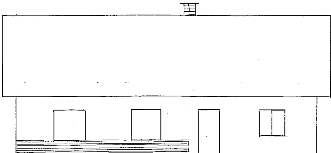
POHLED PŘEDNÍ
